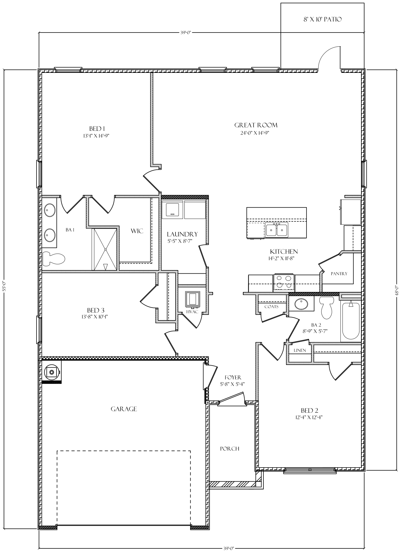
LISMORE - A SCALE: NTS
